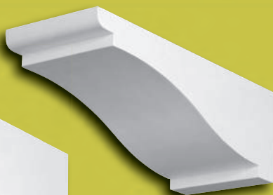
BL 2901 • 18 1/2" Projection • 6 1/4" Height • 7 1/4" Width
